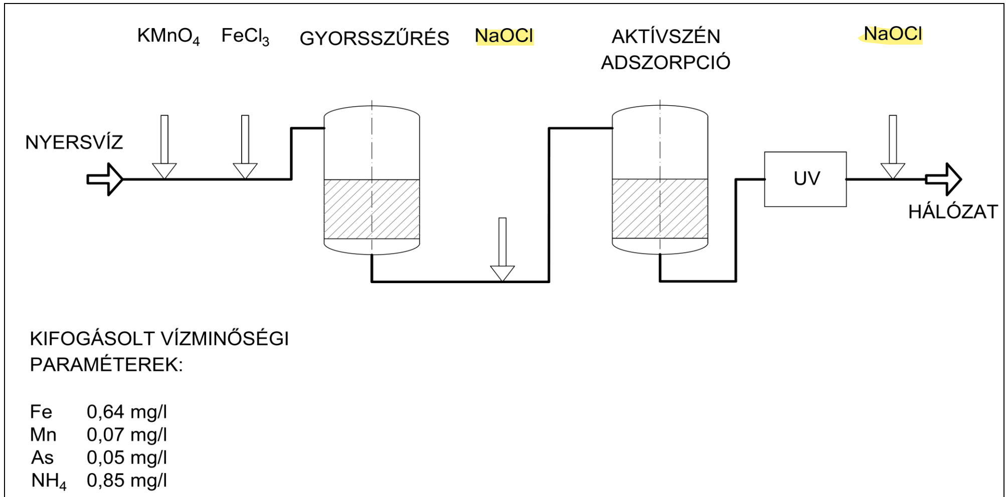
Fe-Mn-As + Törésponti klórozás + UV
